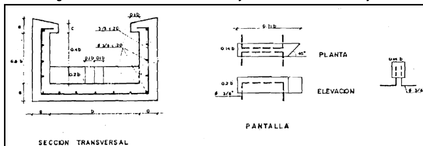
Figura 7-20 Detalle Sección Transversal y Pantalla Estructura de Bajada
