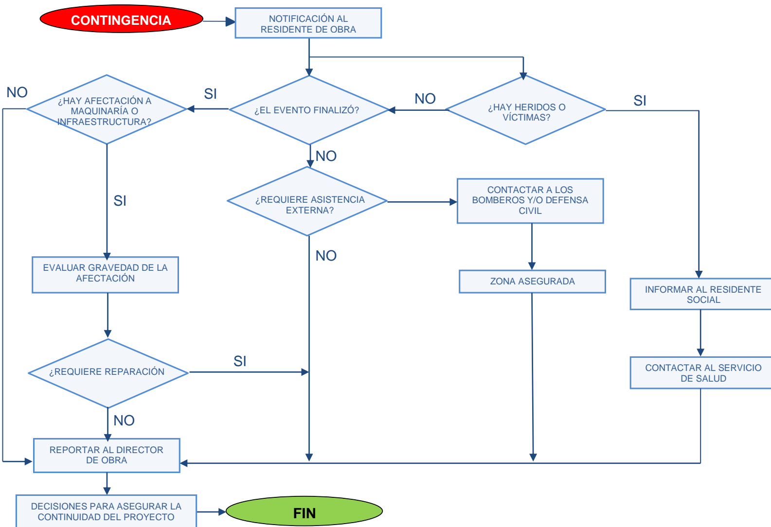
Figura 9-4 Procedimientos de respuesta ante emergencia por sismos
