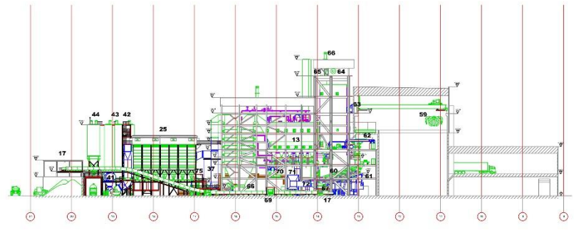
Implantación Sección Longitudinal. Sección C-C
