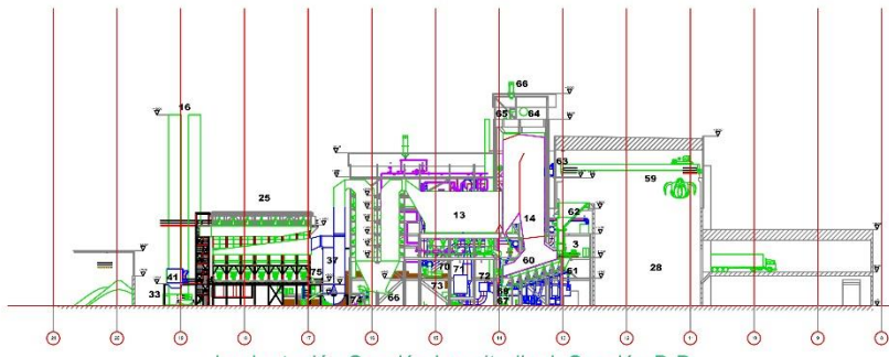
Implantación Sección Longitudinal. Sección B-B
