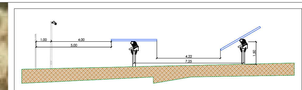
DETALLE DE ESTRUCTURA S: 1/150
